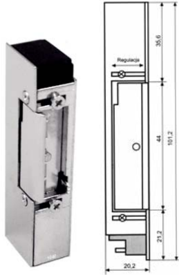
elektrozaczep 12 V z pamięcią electric lock 12 AC with memory
